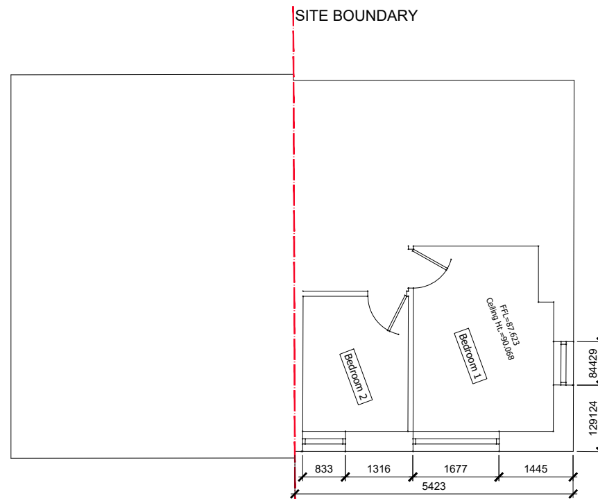
01 EXISTING FIRST FLOOR PLAN PL03 1 : 100
